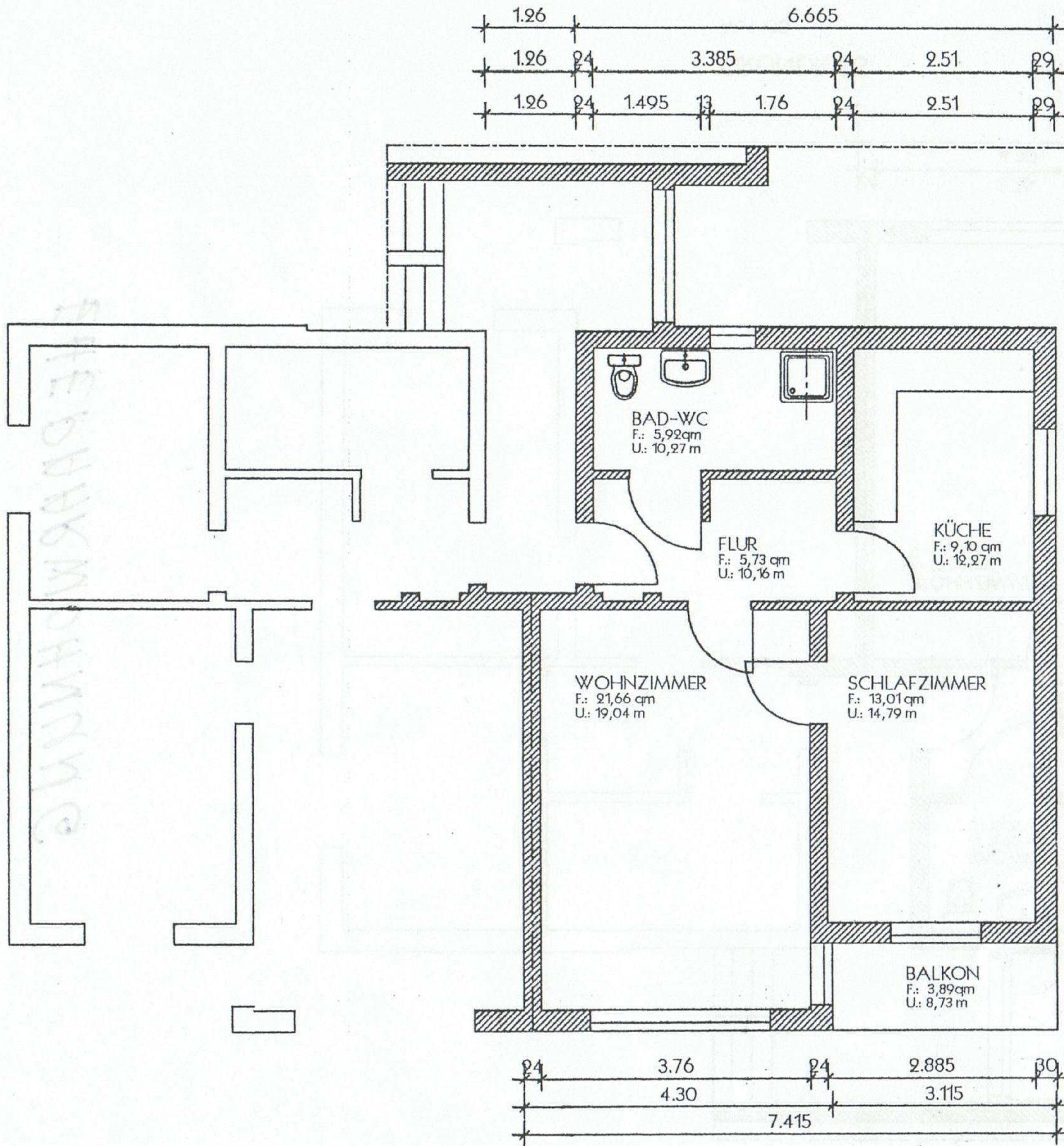
GRUNDRISS M.:1:100
