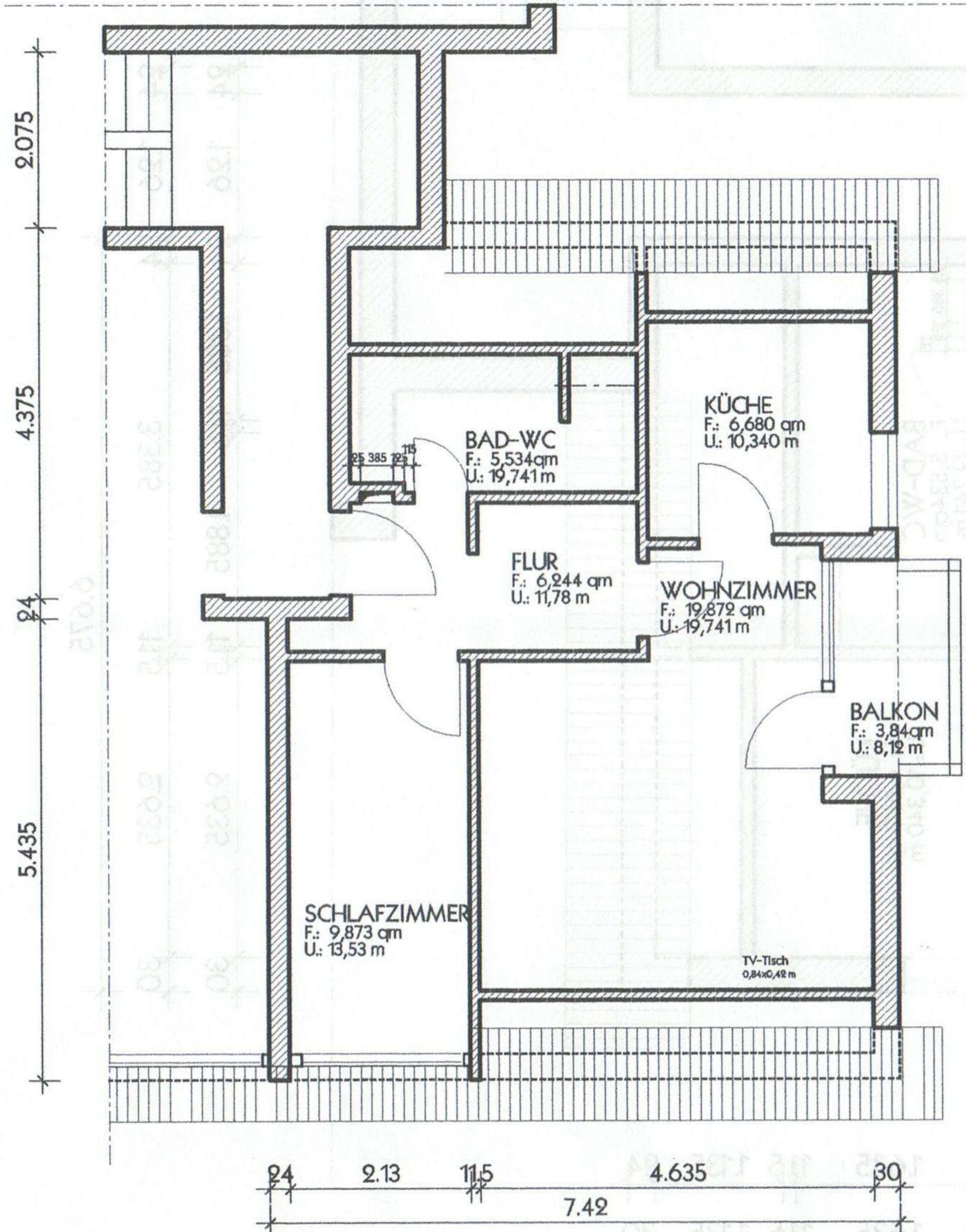
GRUNDRISS M.:1:100
